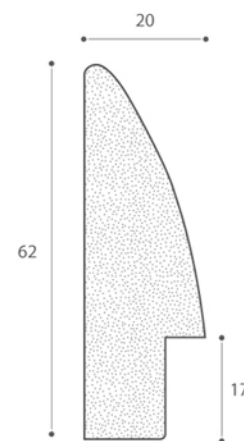
SEZIONE CORNICE SECTION FRAME
