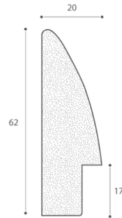
SEZIONE CORNICE SECTION FRAME
